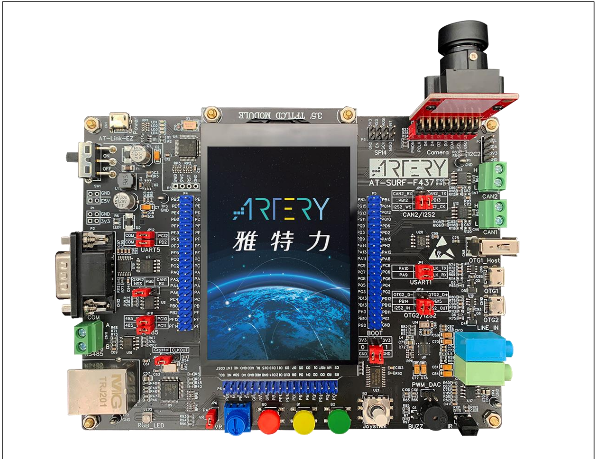
图 1. AT-SURF-F437 V1.x 开发板
